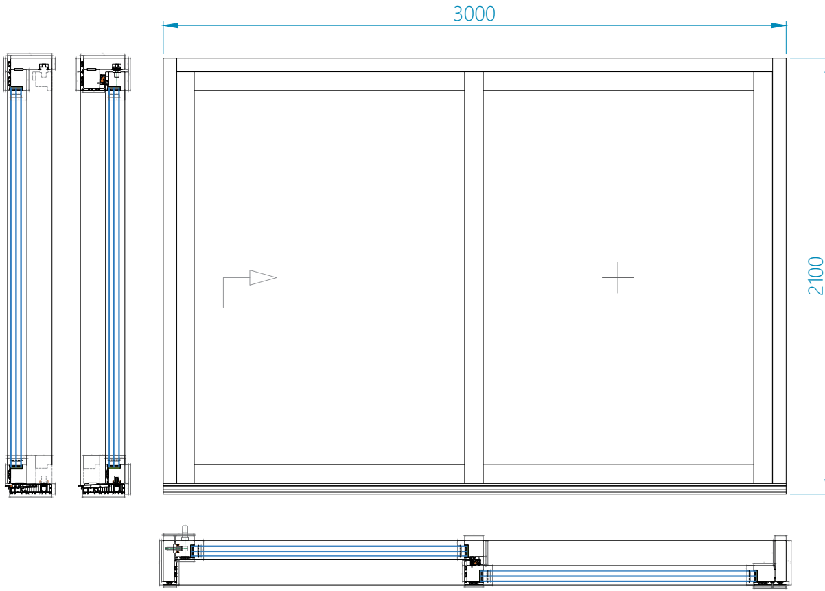
ED199A - ALUCLAD SLIDING DOOR
